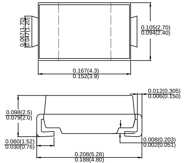
SMA/DO-214AC
