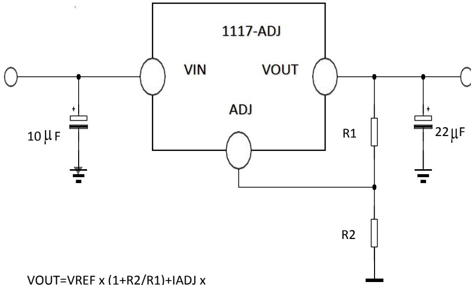
图 2. 典型可调输出电压
